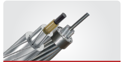
كابلات الكهرباء الهوائية OHTL وأسلاك التآريض OPGW
